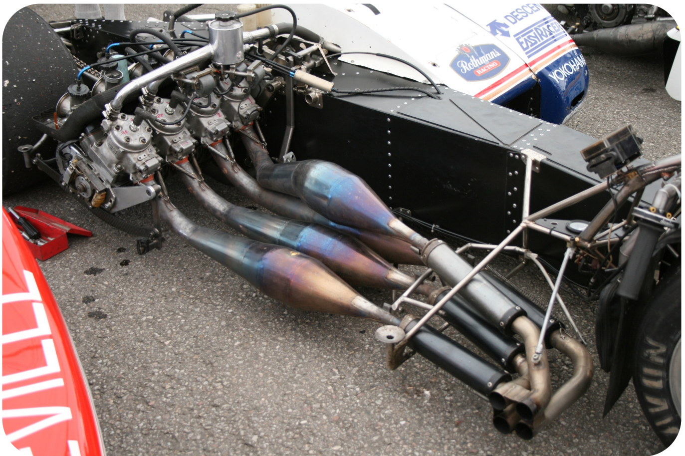
Yamaha TZ750 Motor als Antrieb für ein Gespann mit Resonanzauspuff.
